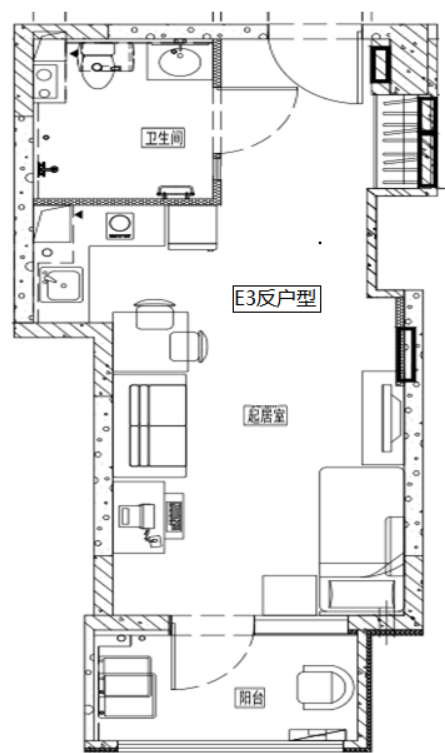
(户型图)
