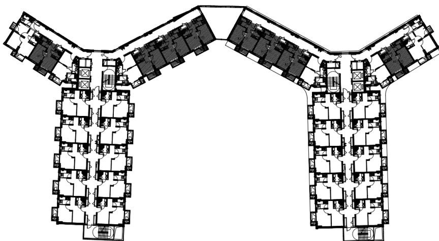
(2#、11#楼 A1 户型分布图)
