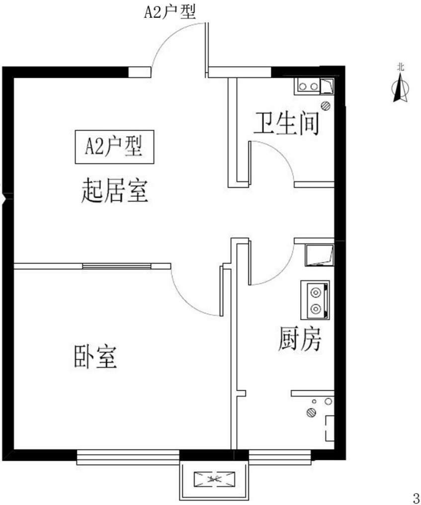
(户型图)
