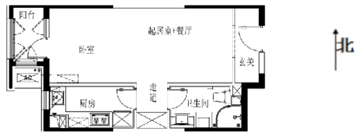
B3户型
