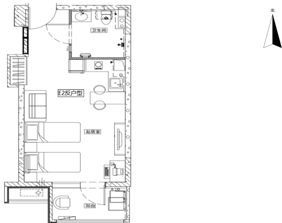
(户型图)
