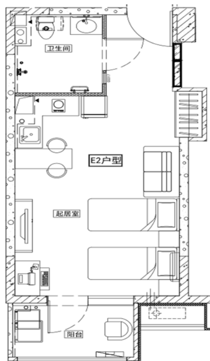
(户型图)
