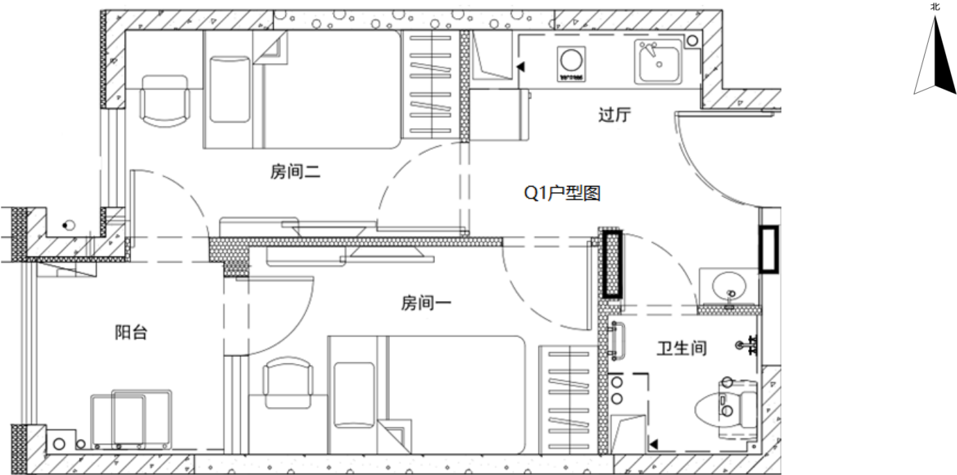
(户型图)
