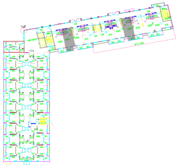
(E2 反户型平面布局图)
