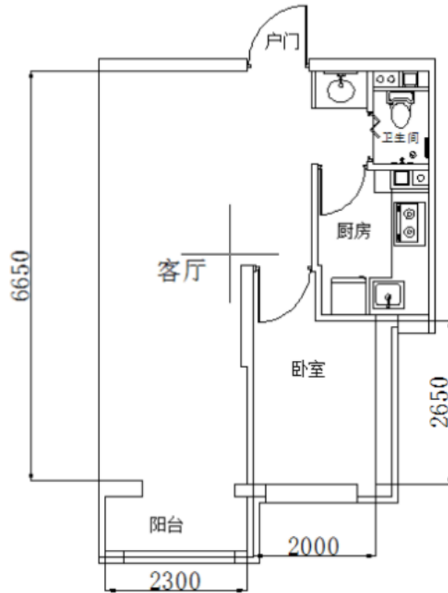
50-A 户型
