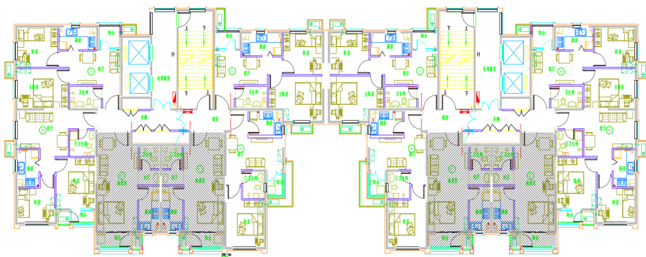
(1-4#楼 C 户型平面布局图)
