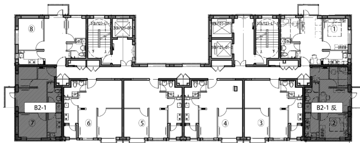
(四区 3 号楼标准层层户型平面布局图)
