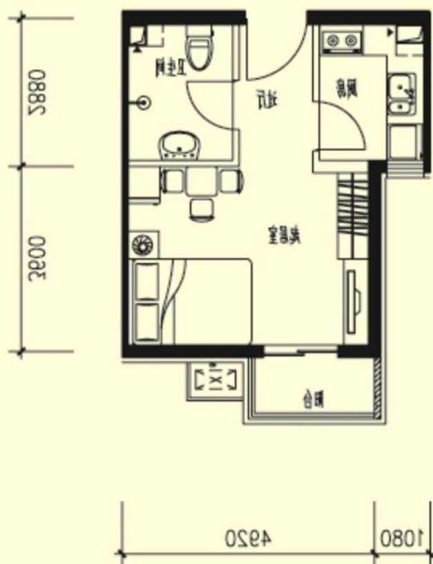
B1反户型图，1室，约33平米
