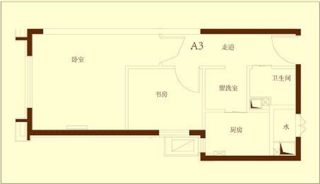
A3 套型： 建筑面积 49.57 平米 / 49.89 平米
