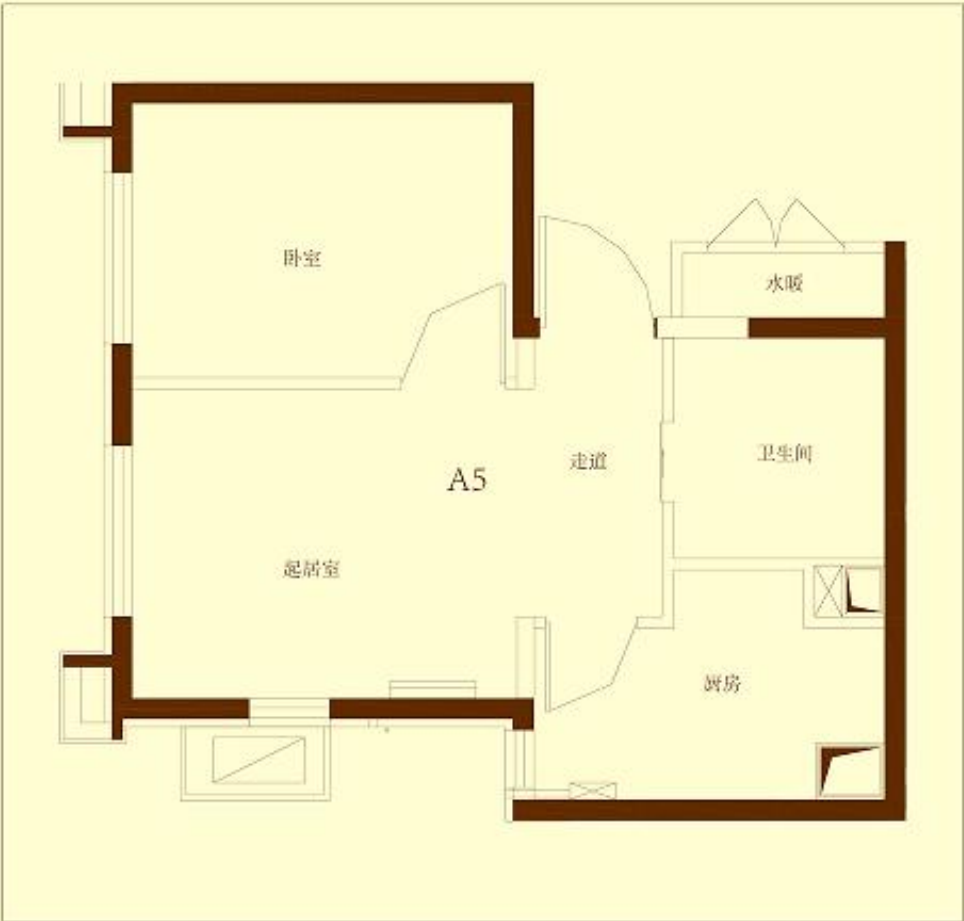
A5 套型：建筑面积 44.62 平米 / 44.74 平米
